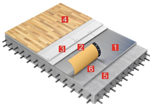
Рис.№2 «Плавающий пол со сборной стяжкой»
