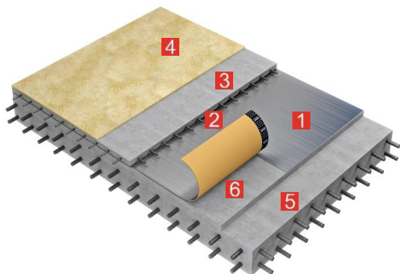
Рис.№1 «Плавающий пол с ц/п стяжкой»
