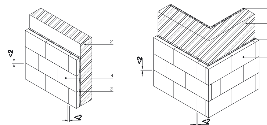
Рисунок 6. Перевязка стыков плит теплоизоляции на внутренних и наружных углах здания
