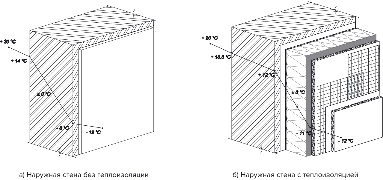
Рисунок 24. Температурная кривая зимой
