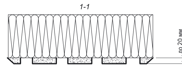
Рисунок 5. Схема точечного нанесения штукатурно-клеевой смеси на плиту
