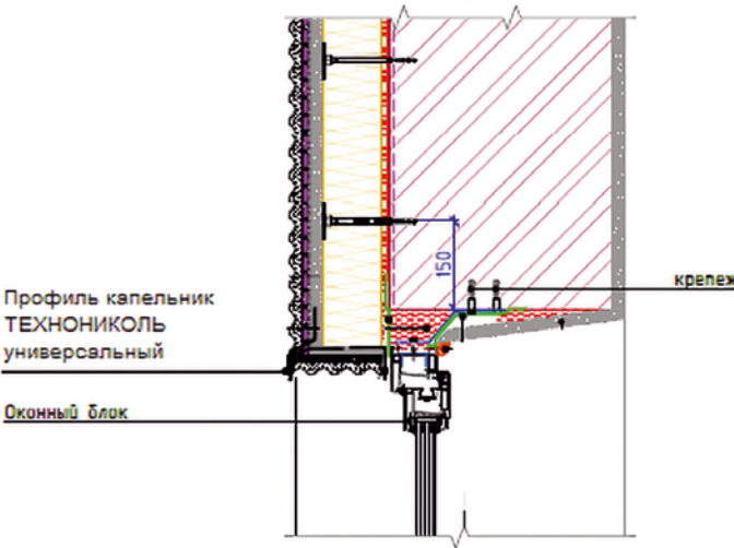
Рисунок 13. Узел расположения капельника над проёмом
