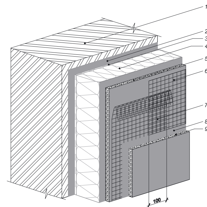
Рисунок 17. Схема соединения двух полотнищ стеклосетки на стене здания
