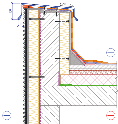
Рисунок 12. Утепление парапета
