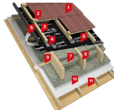
Рис. 6. Строение кровельной системы ТН-ЛЮКСАРД Мансарда
