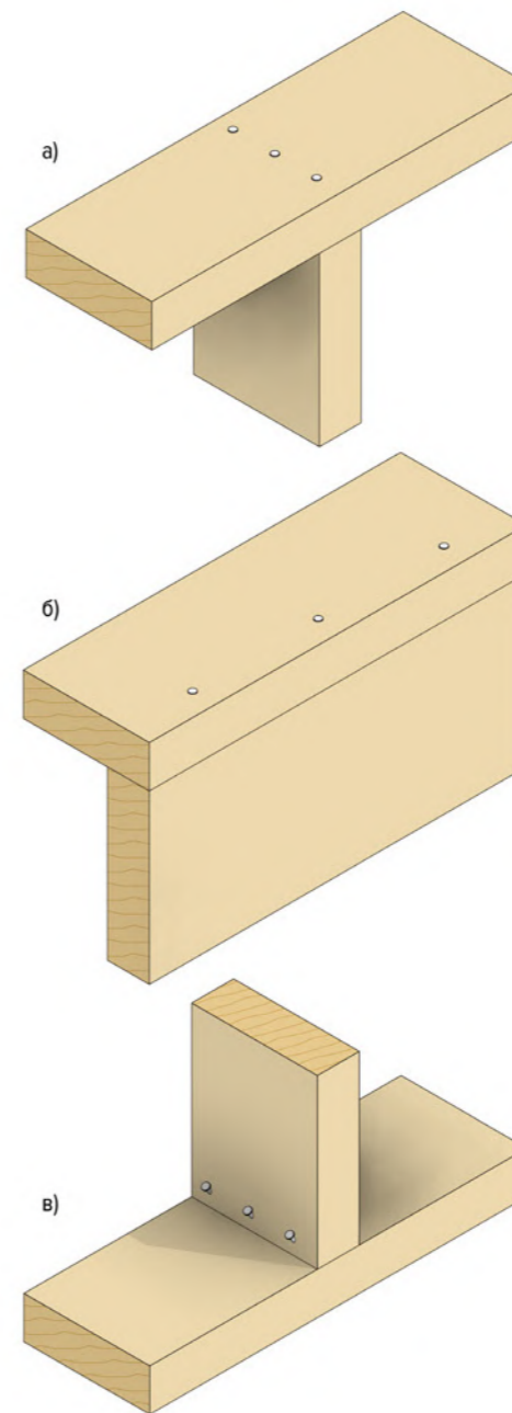
Рисунок 5. Основные соединения
