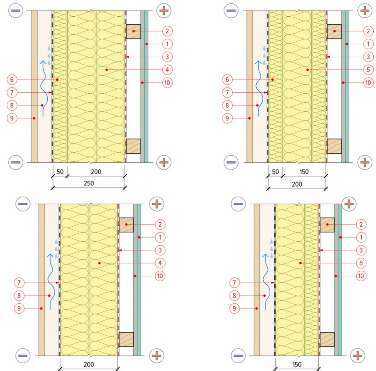
Рисунок 39. Основные варианты теплоизоляции наружных стен
