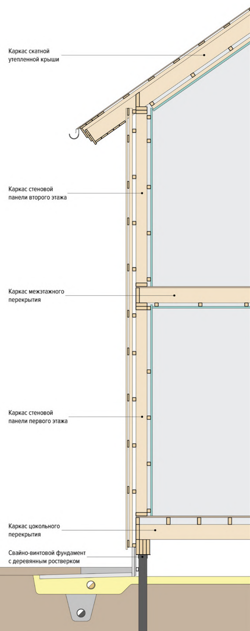
Рисунок 8. Конструкционные разрезы деревянных каркасно-панельных домов по технологии «платформа». Слева - одноэтажный дом с холодным чердаком справа - двухэтажный дом с утепленной мансардой
