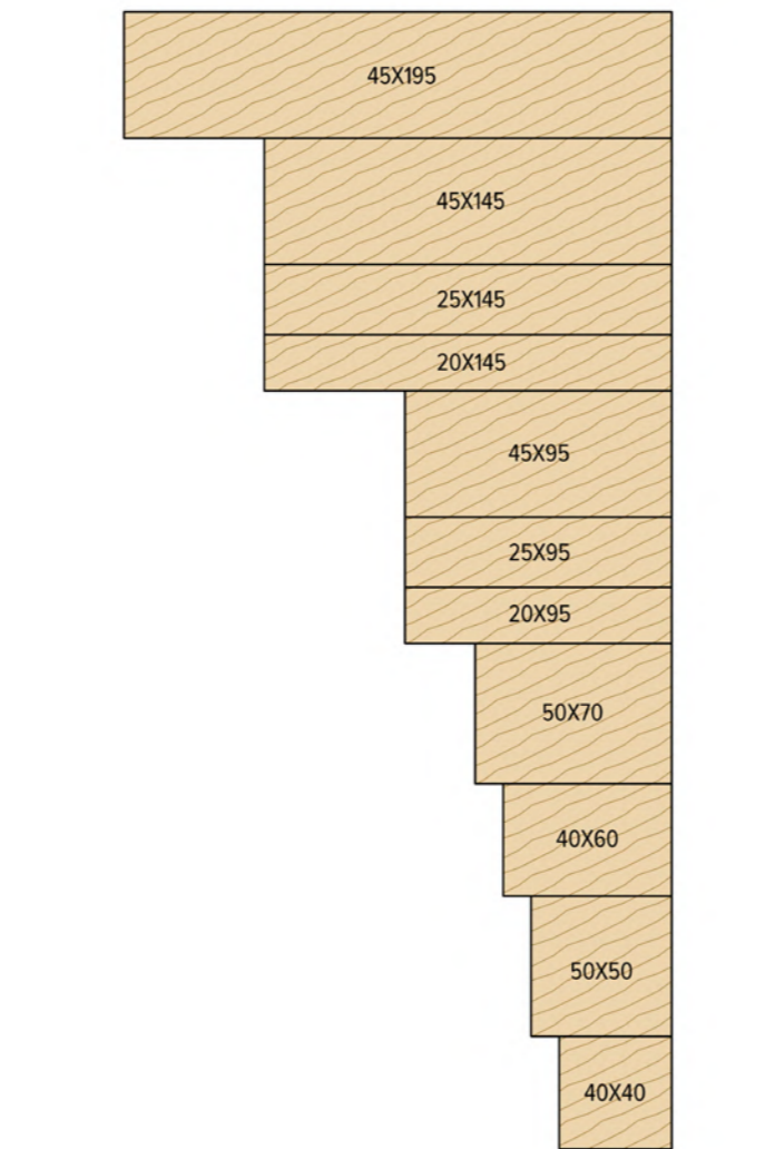
Рисунок 3. Основные сечения калиброванной доски производства ТЕХНОНИКОЛЬ
