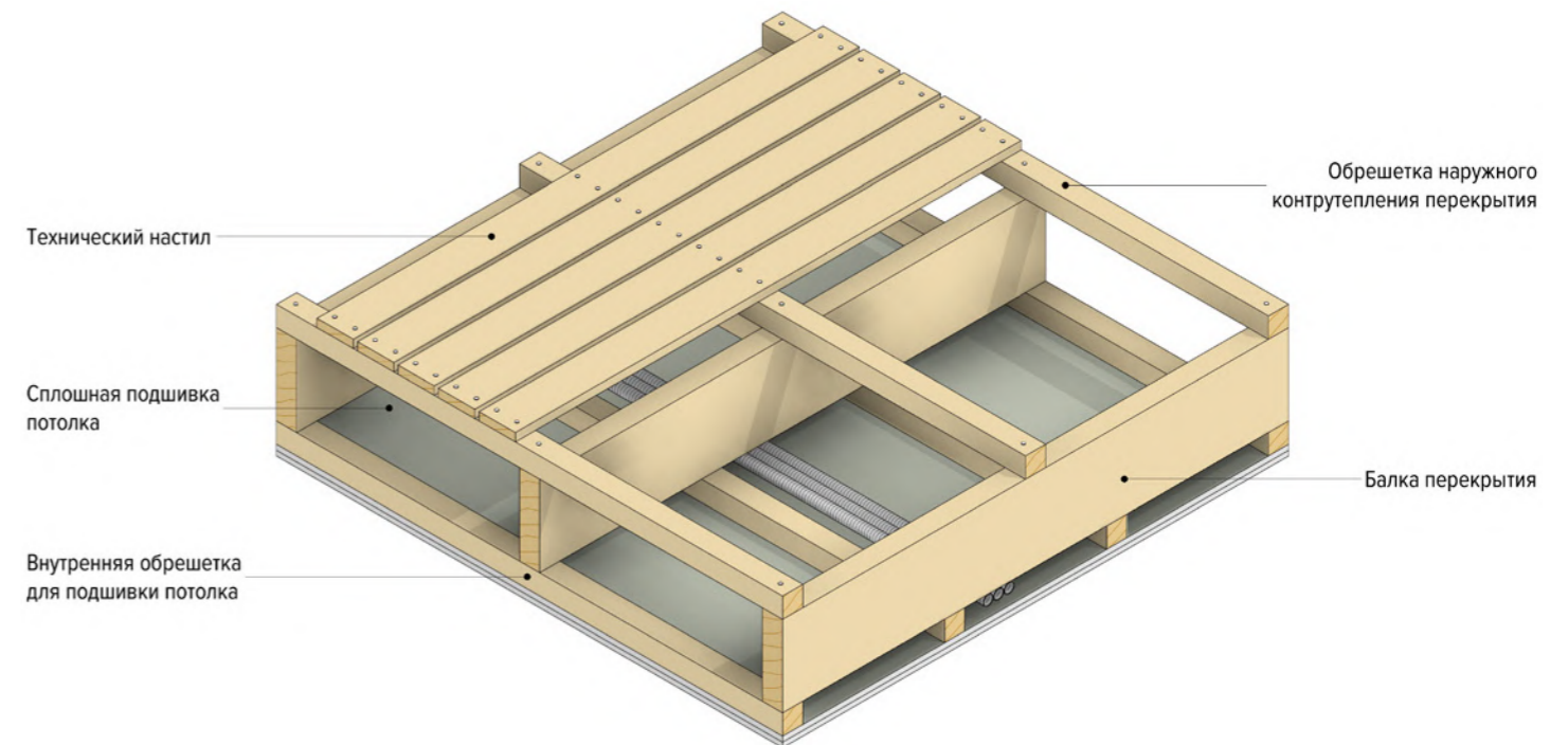
Рисунок 12. Основные конструктивные слои каркаса чердачного перекрытия
