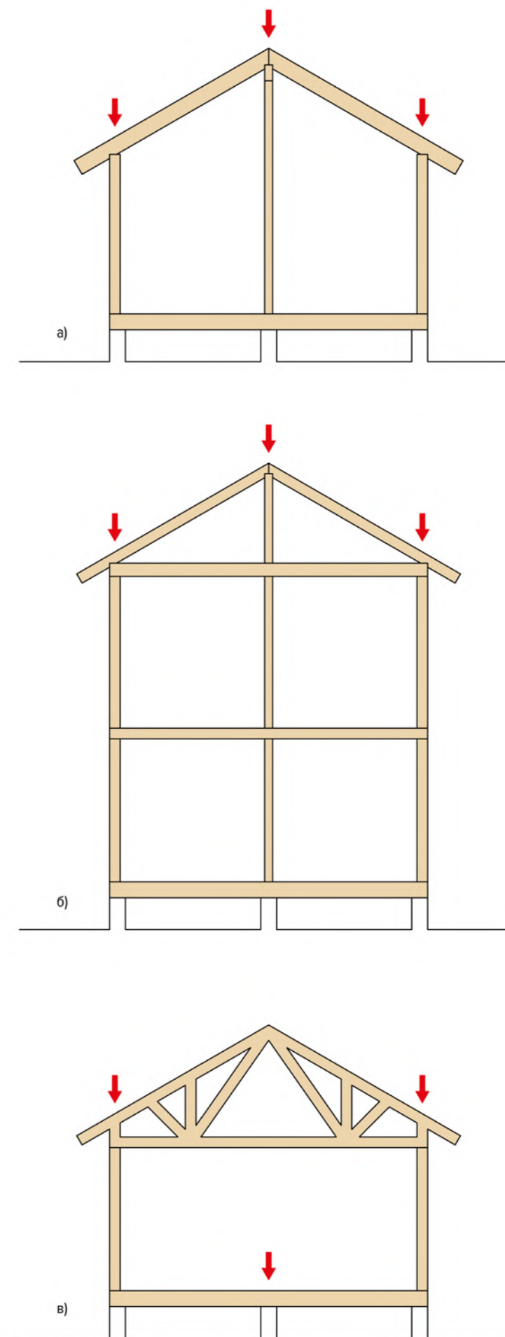
Рисунок 2. Распределение нагрузок а - одноэтажный дом на свайном фундаменте со скатной утепленной крышей; б - двухэтажный дом на свайном фундаменте со скатной неутепленной крышей; в - одноэтажный дом на свайном фундаменте со скатной неутепленной крышей с применением стропильных ферм
