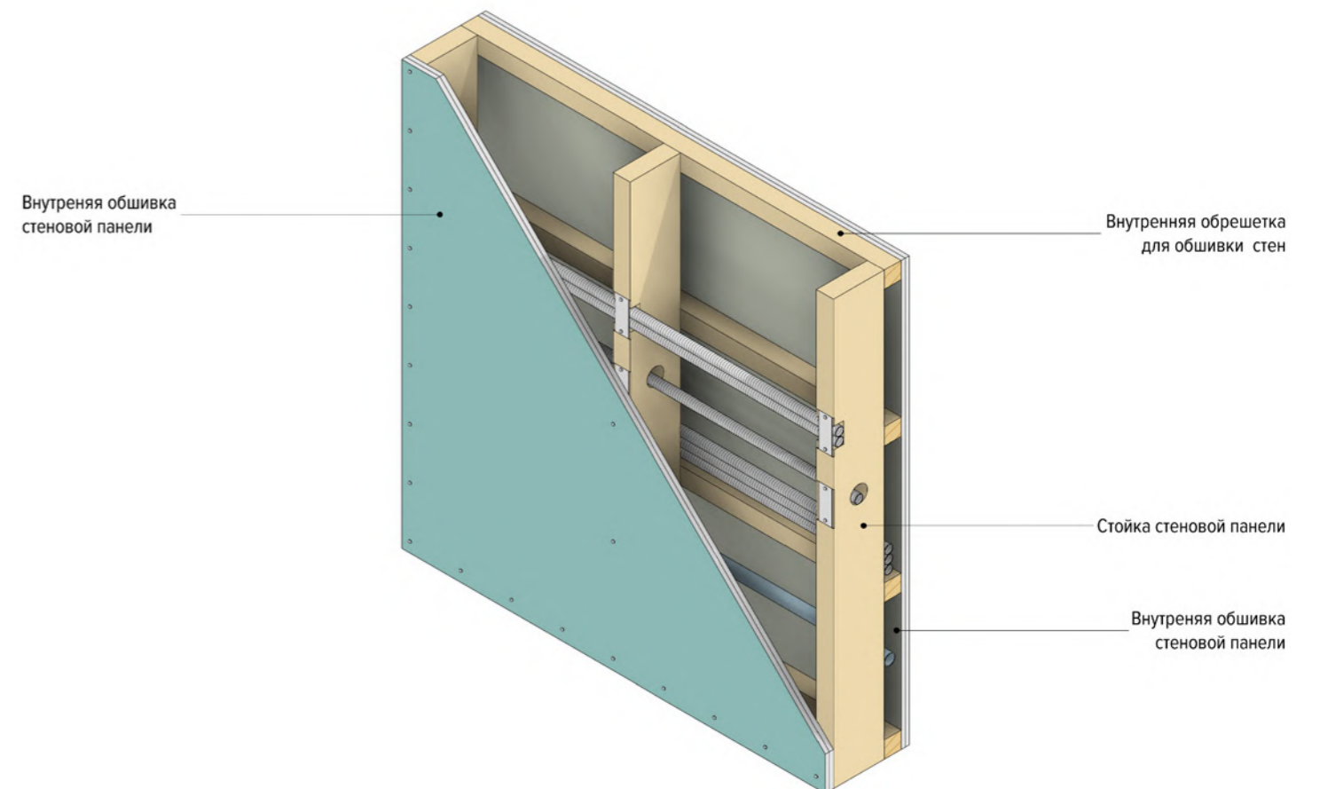
Рисунок 22. Основные конструктивные слои внутренней стеновой панели
